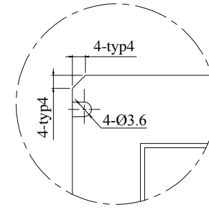
Deatail B 3:1
