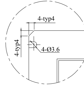
Deatila B 3:1
